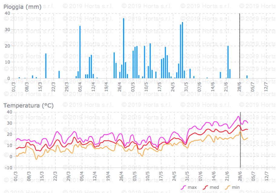
Graf 2: Beležene in predvidene padavine in temperature (na desni strani osi) na slovenskem Krasu. Temperatura(°C) - Temperatura (v °C); Pioggia(mm) - Dež (v mm); med - povprečna; min - najnižja; max - najvišja.
