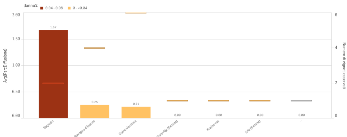
Graf 12: Razširjenost oidija ( Erysiphe necator [Schwein]) glede na občino (%).
