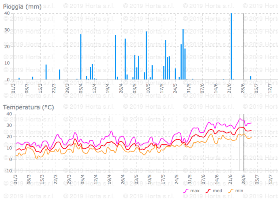
Graf 1: Beležene in predvidene padavine in temperature (na desni strani osi) na italijanskem Krasu . Temperatura(°C) - Temperatura (v °C); Pioggia(mm) - Dež (v mm); med - povprečna; min - najnižja; max - najvišja.
