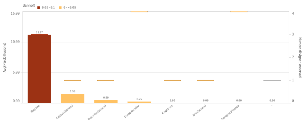
Graf 13: Razširjenost Black Rot Guignardia bidwellii (Ell.) na občino (v %)
